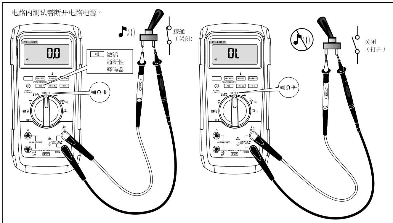
图 4.通断性测试
