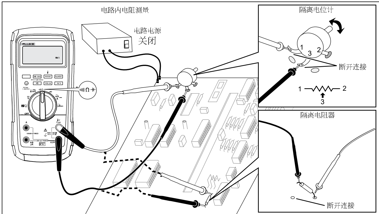
图 5.电阻测量
