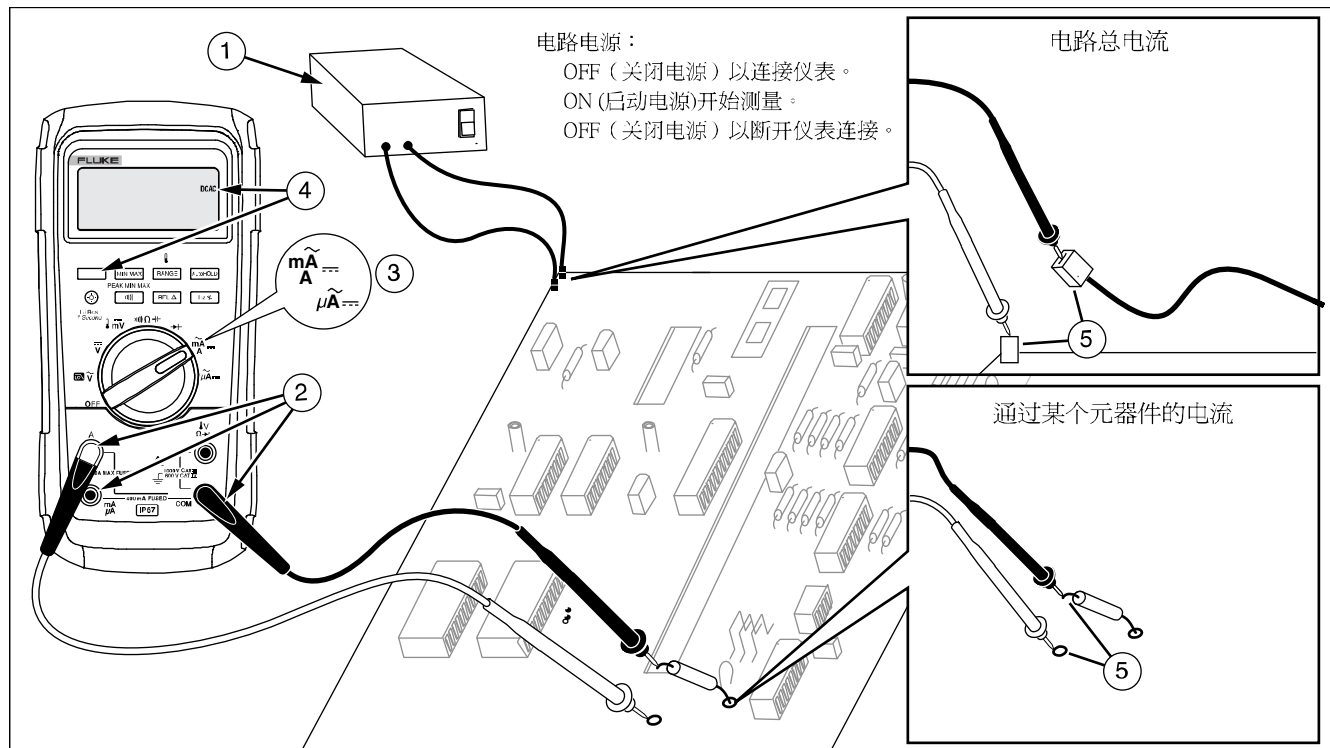
图 8. 电流测量
