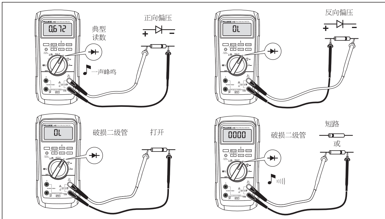
图 7.二极管测试
